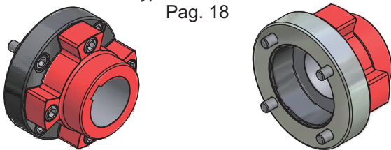
Giunto elastico per fissaggio a parete con mozzo esterno "V" Flexible coupling for flange connection with external "V" hub
