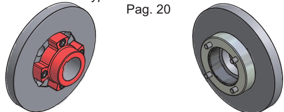
Giunto elastico per fissaggio a parete con Disco Freno "PA" Flexible coupling for flange connection with Brake Disc "PA"
