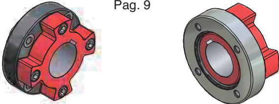
Giunto elastico con mozzo incassato "U" Flexible coupling with internal "U" hub
